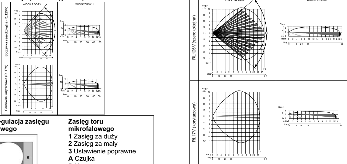
Rysunek 4. Charakterystyki detekcyjne czujek iWISE DT AM
